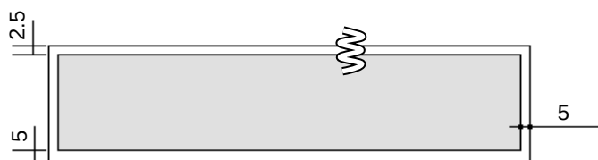
【裏面かぶり寸法】
