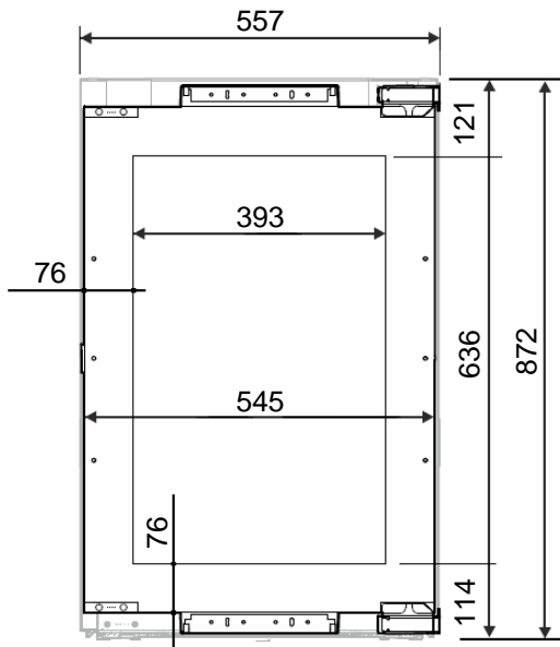
【本体ドアフレーム詳細寸法】
