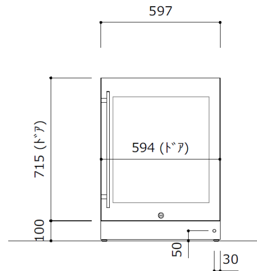
正面図
