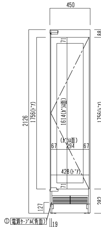
正面図
