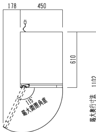
平面図
